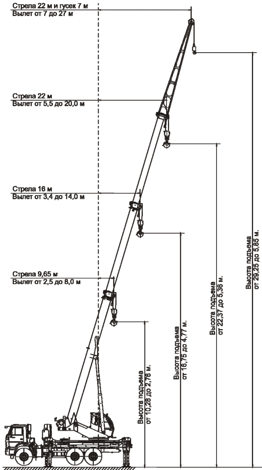
Рисунок 1 – Общий вид крана в рабочем положении с гуськом 7 м
