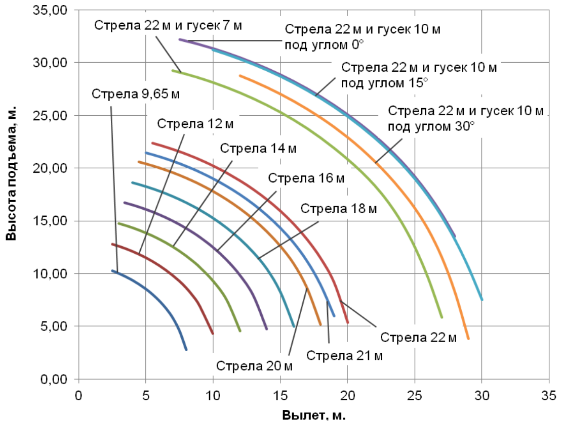
Рисунок 17– Высота подъема крюка
