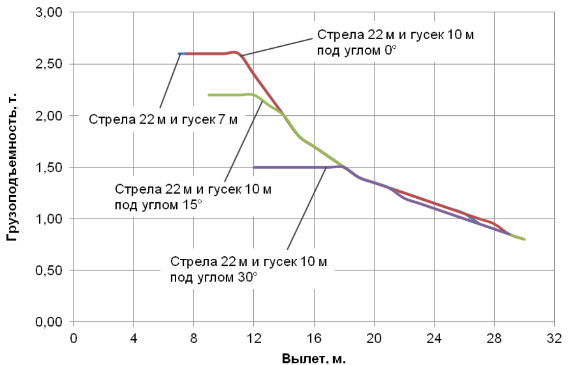
Рисунок 16 – Грузовые характеристики на стреле с гуськом с противовесом 5,4 т. Зона работы 360°. Полный опорный контур
