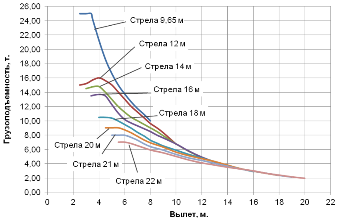
Рисунок 15 – Грузовые характеристики на стреле с противовесом 5,4 т. Зона работы 360°. Полный опорный контур
