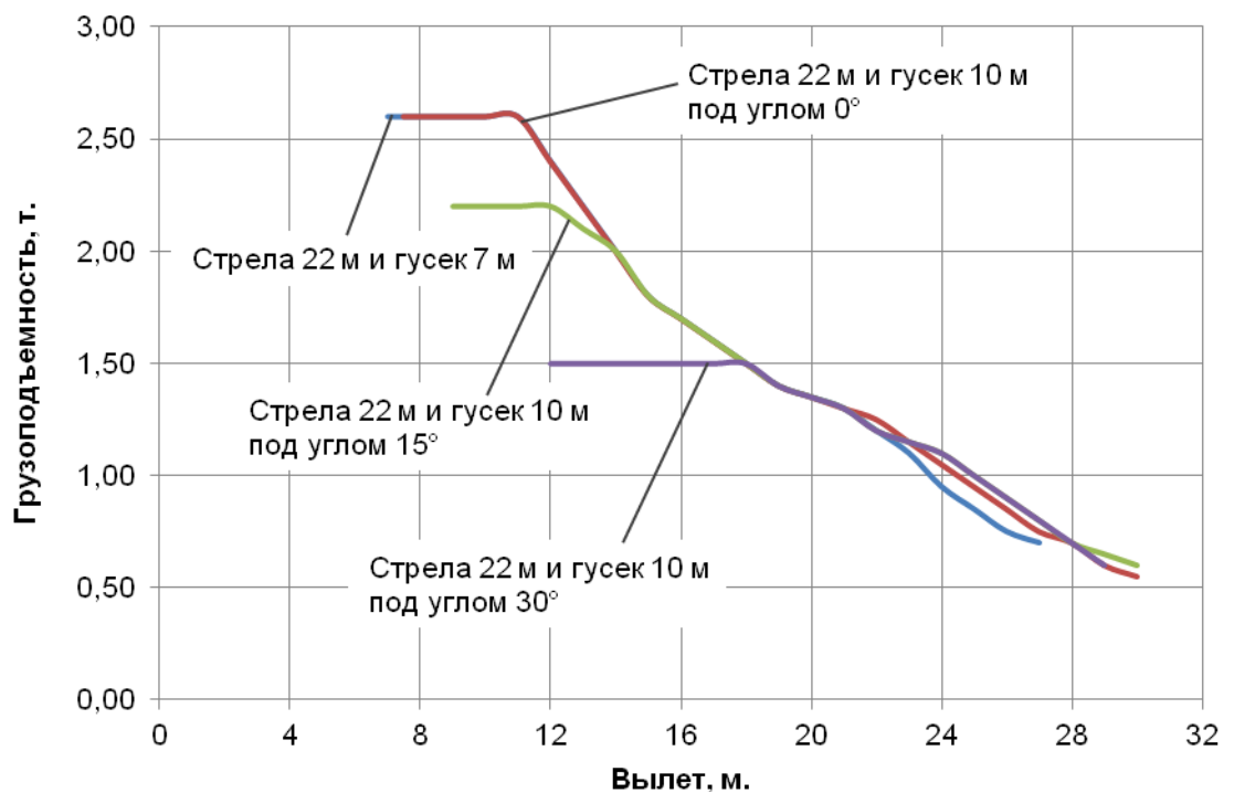
Рисунок 13 – Грузовые характеристики на стреле с гуськом с противовесом 4 т. Зона работы 360°. Полный опорный контур
