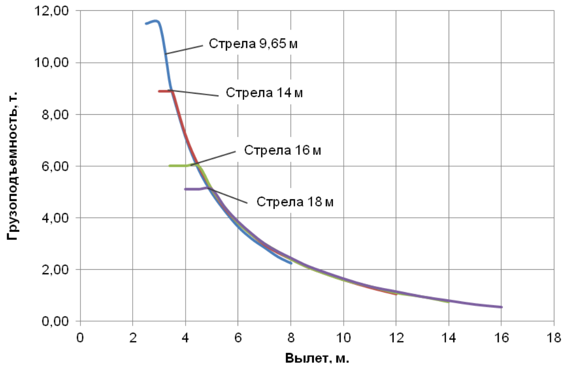
Рисунок 14 – Грузовые характеристики на стреле с противовесом 4 т. Зона работы 360°. Неполный опорный контур
