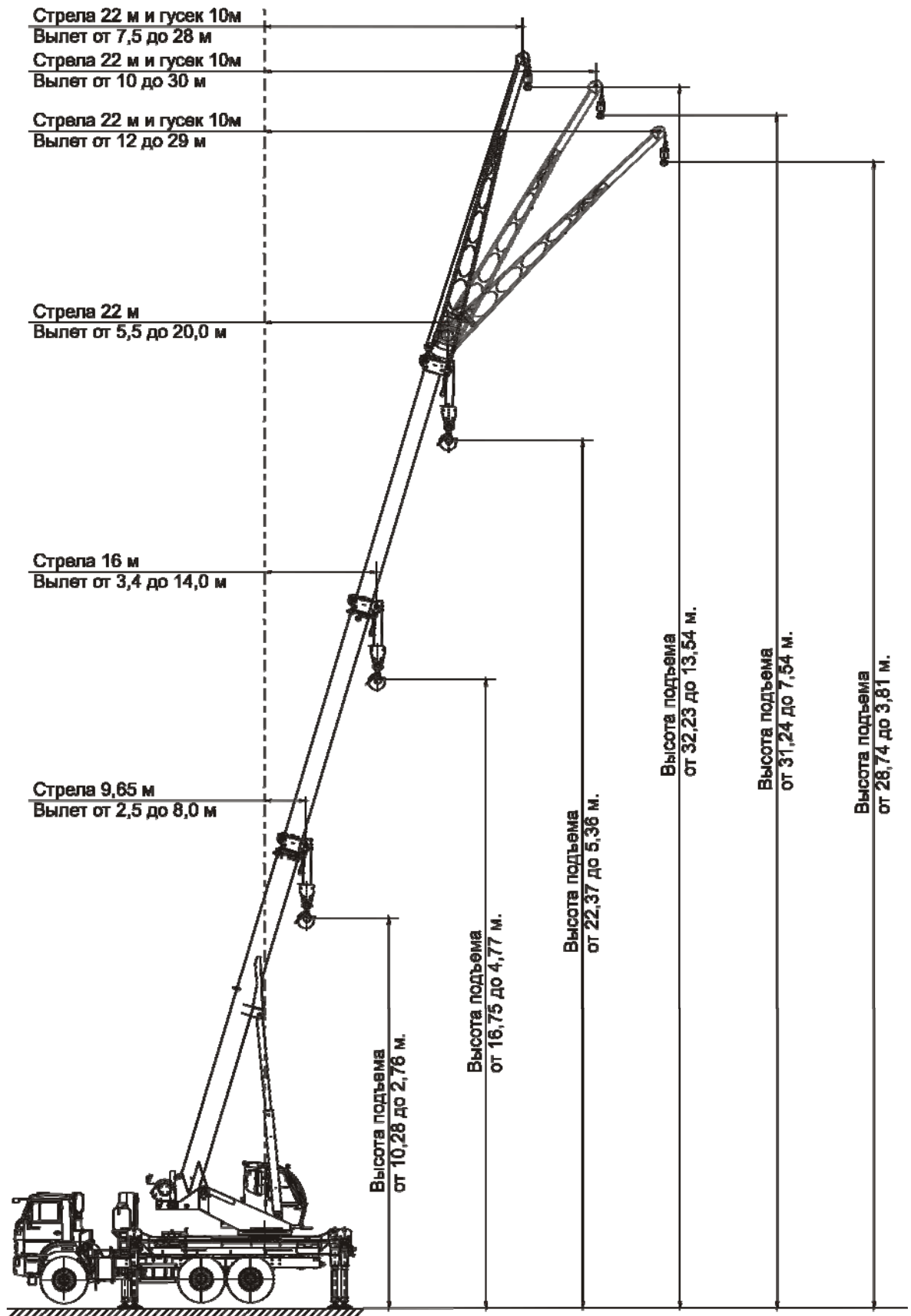
Рисунок 2 – Общий вид крана в рабочем положении с гуськом 10 м.
