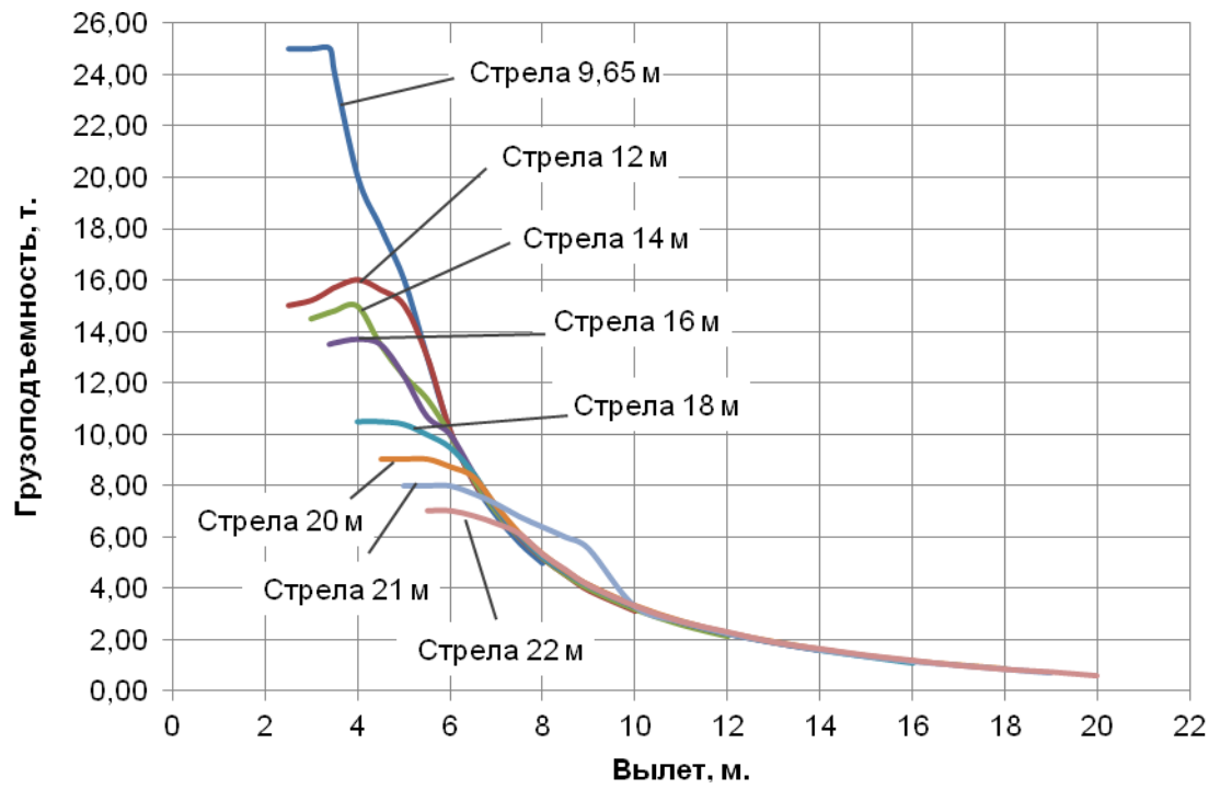
Рисунок 10 – Грузовые характеристики на стреле с противовесом 1 т. Зона работы 360°. Полный опорный контур
