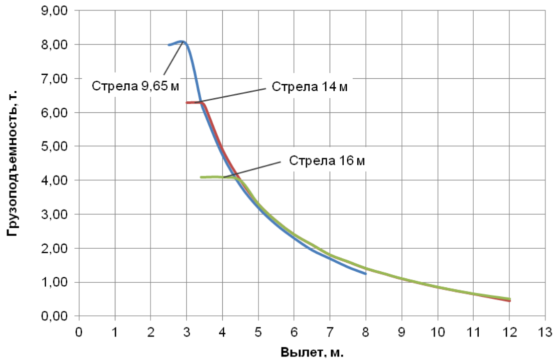
Рисунок 11 – Грузовые характеристики на стреле с противовесом 1 т. Зона работы 360°. Неполный опорный контур
