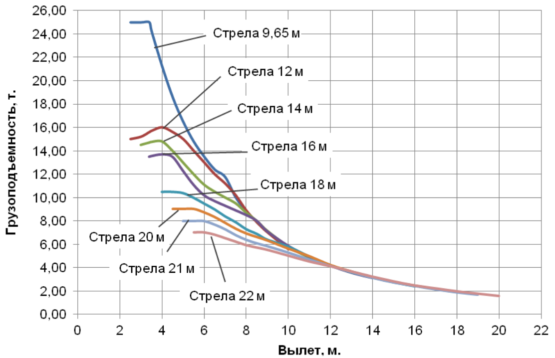
Рисунок 12 – Грузовые характеристики на стреле с противовесом 4 т. Зона работы 360°. Полный опорный контур
