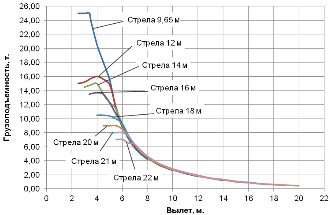
Рисунок 6 – Грузовые характеристики на стреле без противовеса Зона работы 360°. Полный опорный контур
